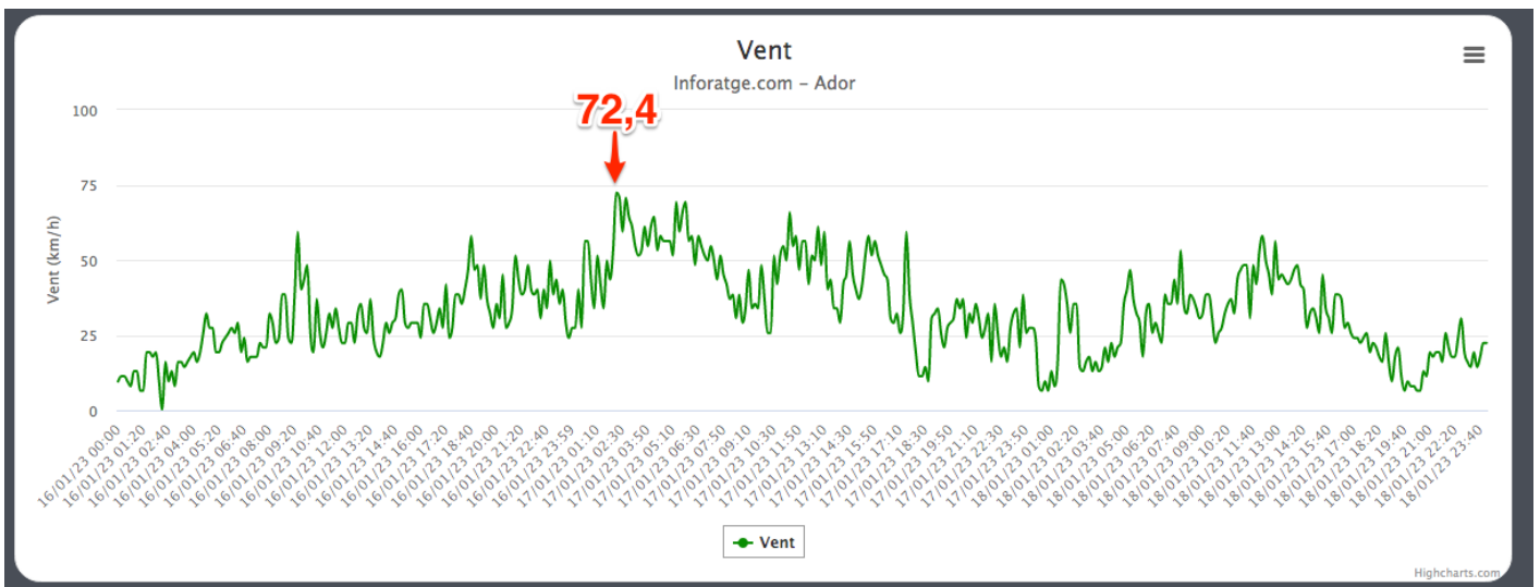
Ráfagas de viento registradas en ADOR entre el 16 y el 18/01/23 https://inforatge.com/meteo-ador
